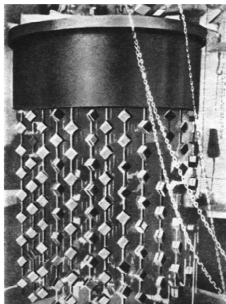
v nedokončeném atomovém reaktoru v Heigerlochu našla skupina Alsos kostky uranu, zavěšené na olověném víku reak- toru, ponořené do těžké vody
